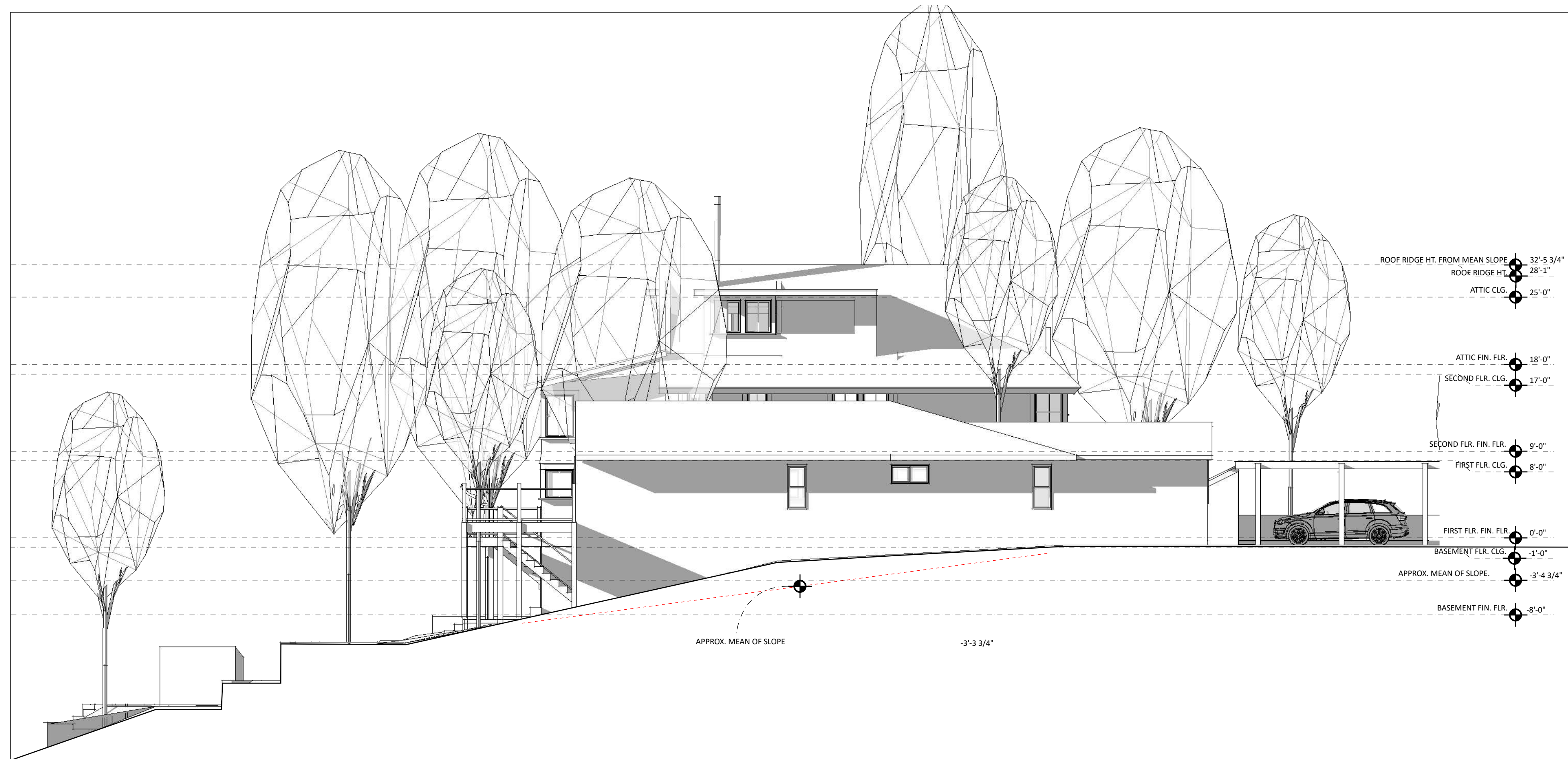
1 N - ELEVATION SCALE: 1/8" = 1' - 0"
