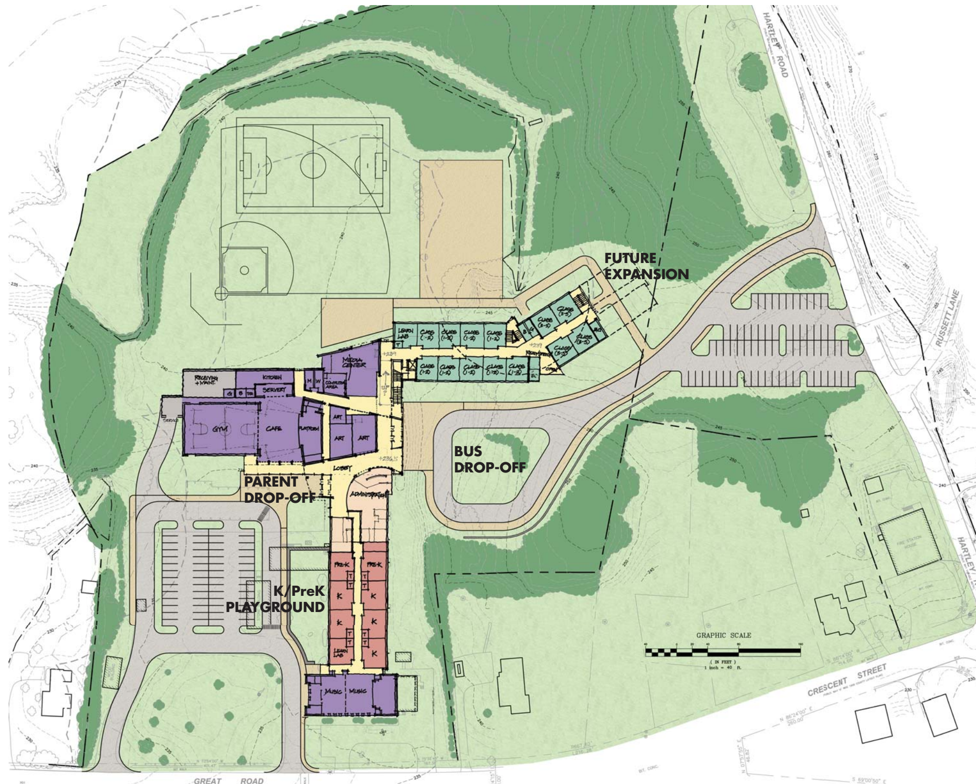
SITE PLAN OPTION D
